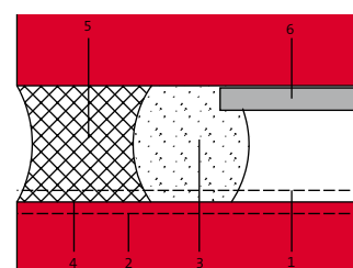
◀ Dehnungsfuge Ausbildung vertikal und horizontal: 1. Fuge gestaut 2. Fuge gedehnt 3. Schaumstoffprofil 4. Haftgrundierung 5. Fugendichtstoff 6. Konsolanker © Halfen
